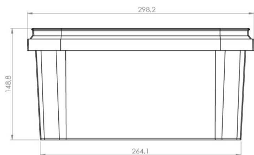
Wiadro 5 litrowe Pr Wiadro- 350/5Pr Pokrywka – 350/PR
